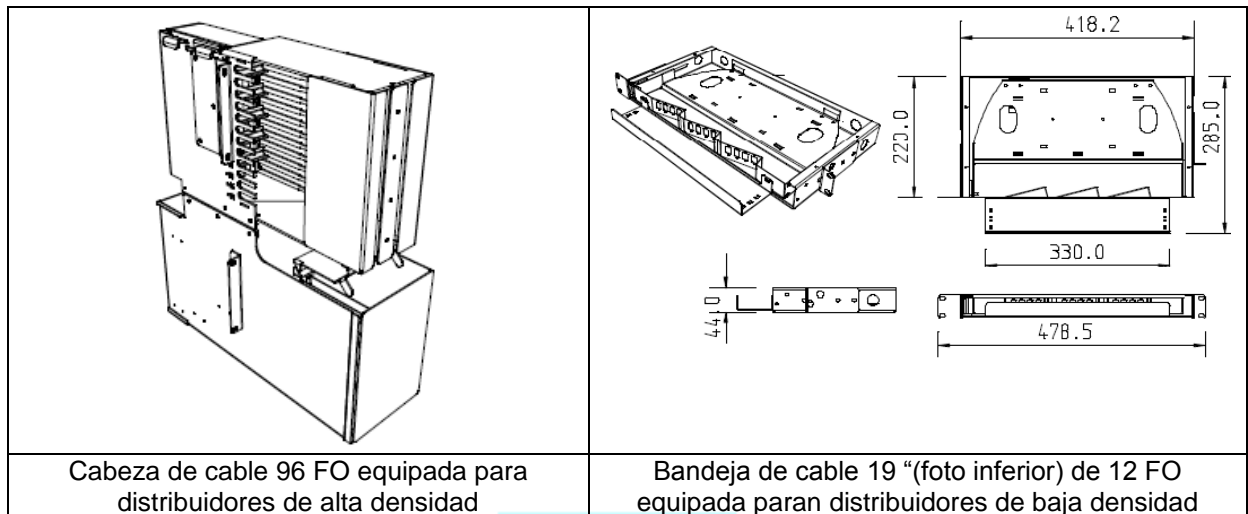
Figura Nro. 4. ilustrativa de rack y cabeza/ bandeja de FO para distribuidor de alta y baja densidad respectivamente.
