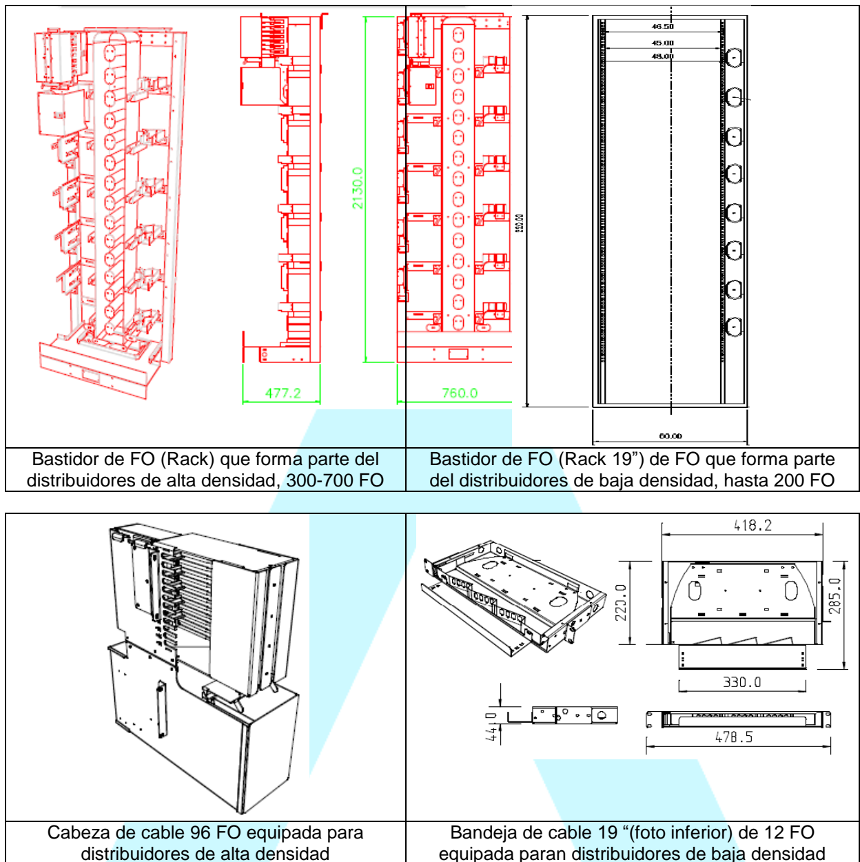
Figura Nro. 4. ilustrativa de rack y cabeza/ bandeja de FO para distribuidor de alta y baja densidad respectivamente.
