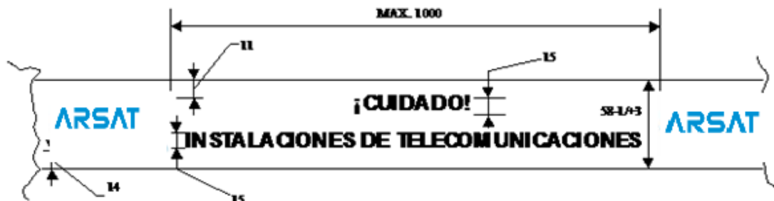
Figura Nro. 6. Cinta de advertencia. Ejemplo.
